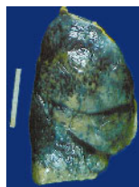
70歳 1日60本 55年
